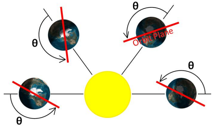
Figure 2: Órbita heliosincrónica con condiciones de iluminación solar constante.
