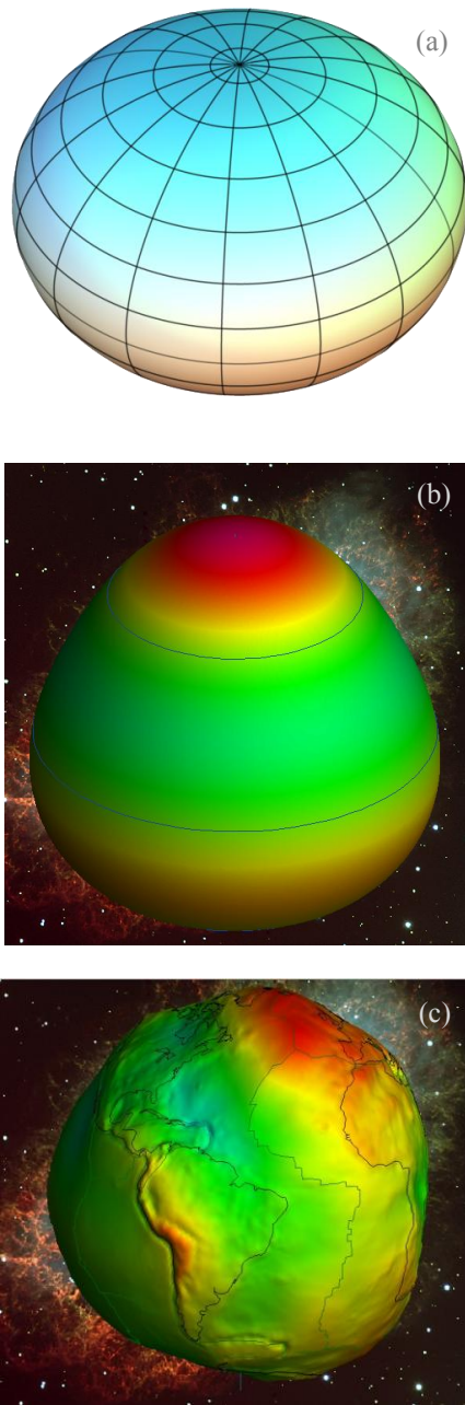
Figura 1: (a) Representación visual del armónico zonal J2, (b) representación visual del armónico zonal J3 y (c) Modelo Geopotencial tomando en cuenta los diferentes armónicos (zonales, sectoriales y teserales).
