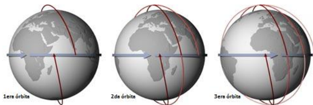
Figura 3: Ilustración del periodo de revisita de una órbita heliosincrónica
